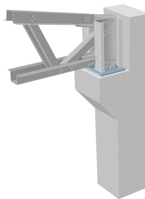
KÍBOVÝ PRÍPOJ NA ŽELEZOBETÓNOVÝ STĽP
